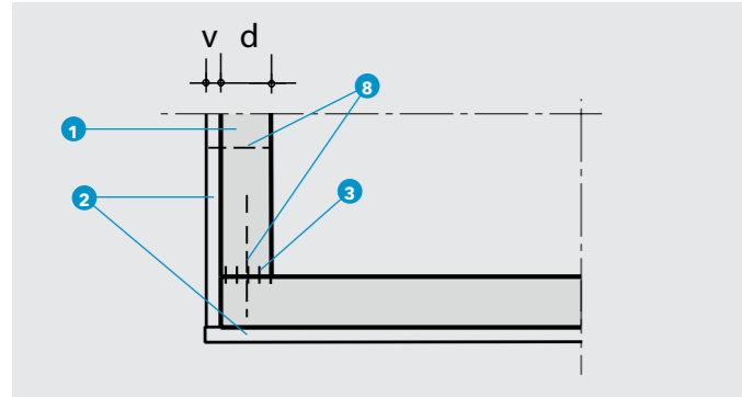
DETTAGLIO P - COLLEGAMENTO AL SOLAIO - SEZIONE TRASVERSALE
