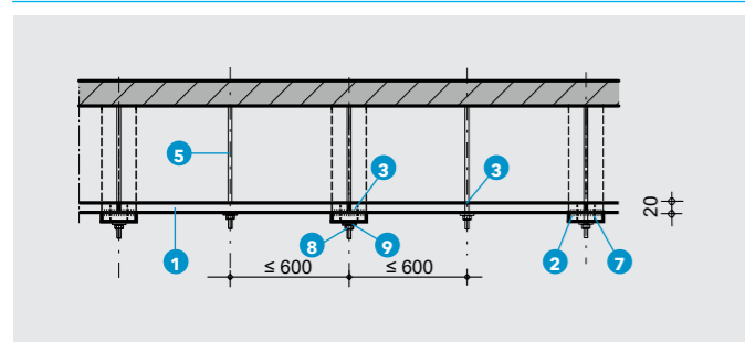
DETTAGLIO N - SEZIONE LONGITUDINALE
