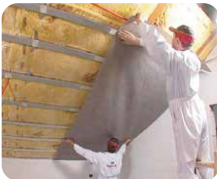
Slika 7: Na C-profil pritrdimo parno oviro z dvostranskim lepilnim trakom
