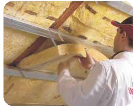
Slika 6: Pod kovinski C-profil vstavimo drugi sloj izolacije
