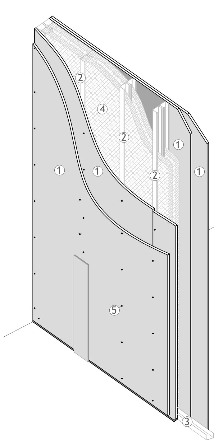
ISOMETRICA
