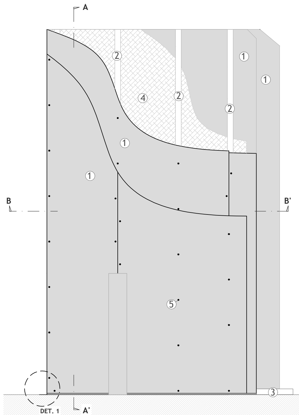
ELEVACION
