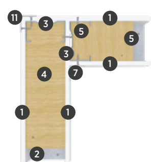
* Detalle 3: Encuentro en L
