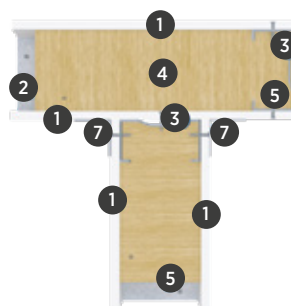
* Detalle 2: Encuentro en T
