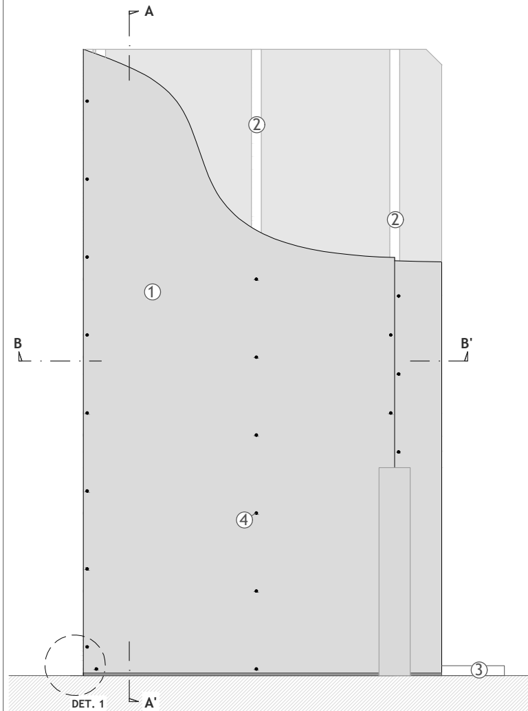
ELEVACION
