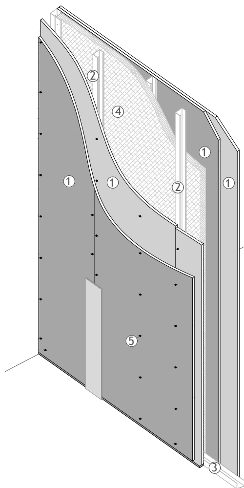
ISOMETRICA
