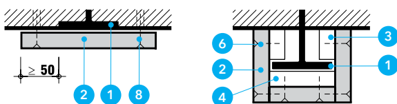
Detal C - Obudowa jednostronna
