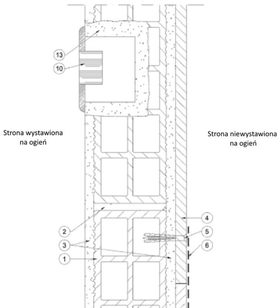
Ilustracja A.2.2.7.4 Zbliżenia fragmentów ocenianej instalacji
