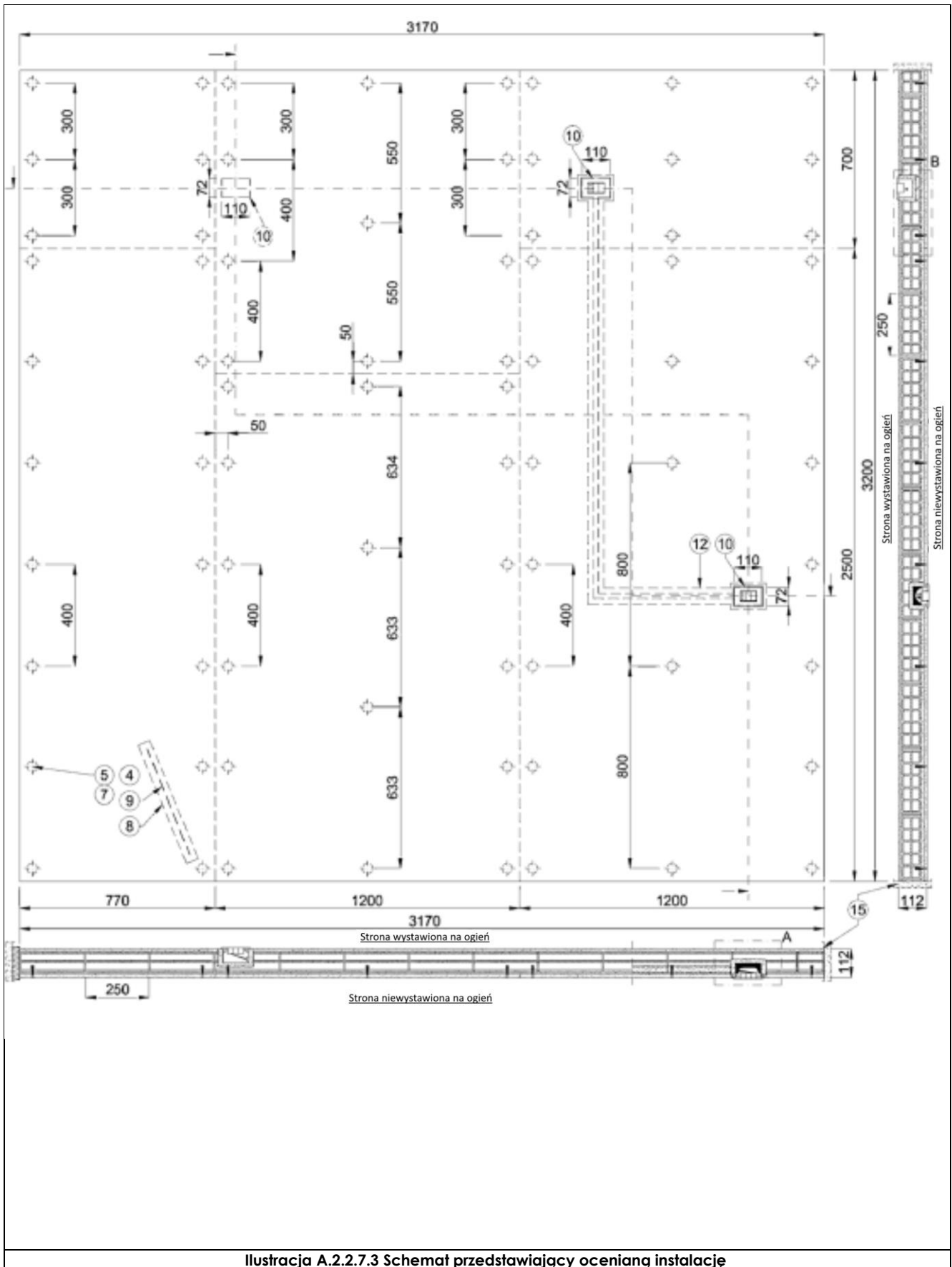
Ilustracja A.2.2.7.3 Schemat przedstawiający ocenianą instalację
