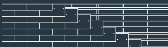
Pose à pureau horizontal
