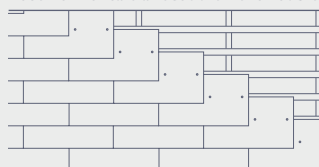
Recouvrement double
