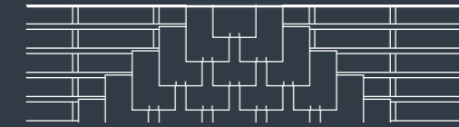
Pose à claire-voie à recouvrement double
