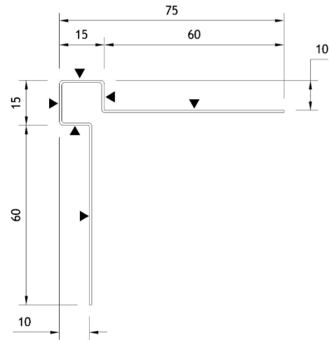
EQUITONE aansluitprofiel/raam Art. N° 4031226
