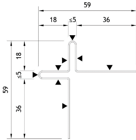
EQUITONE voegprofiel met rib voor horizontale voeg Art. N° 4031409
