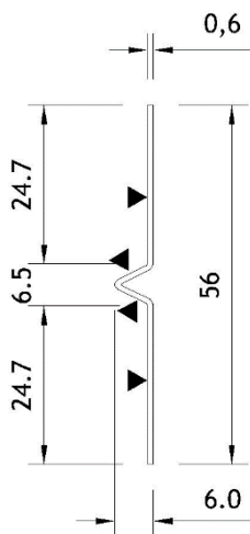
EQUITONE voegprofiel met rib voor horizontale voeg Art. N° 4031409
