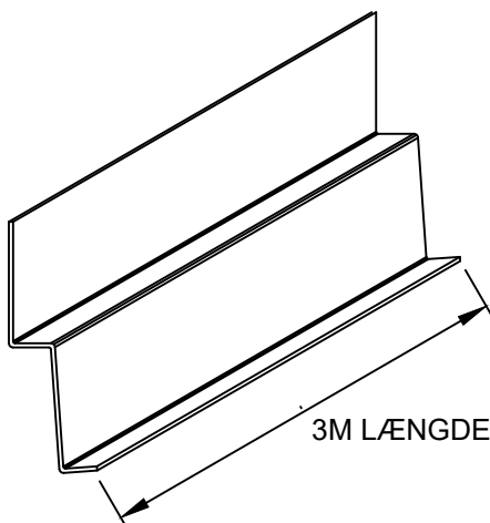
SEKTION STARTPROFIL 1:1
