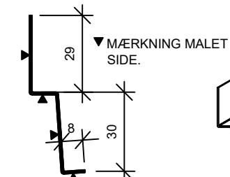
STARTPROFIL
