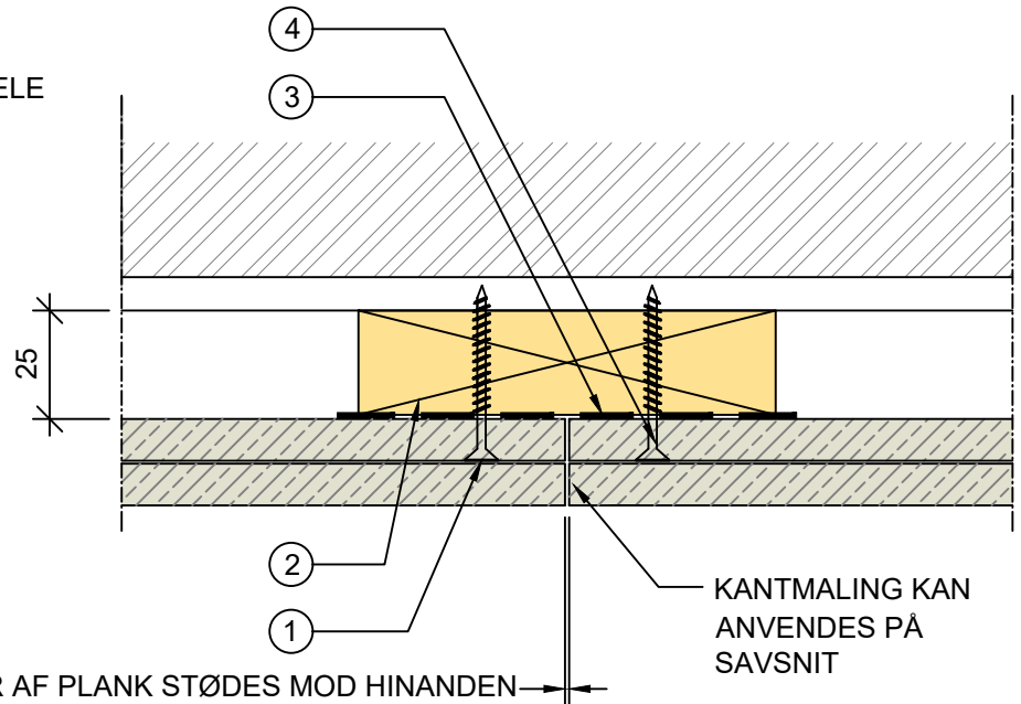
SAMMENFALDENE FUGER PLAN 1:2
