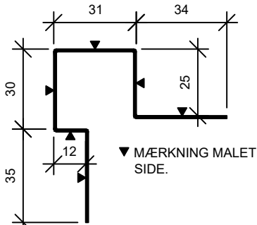
ASYMMETRISK UDVENDIGT HJØRNE PROFIL
