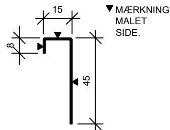
ENKEL ENDEKANT PROFIL
