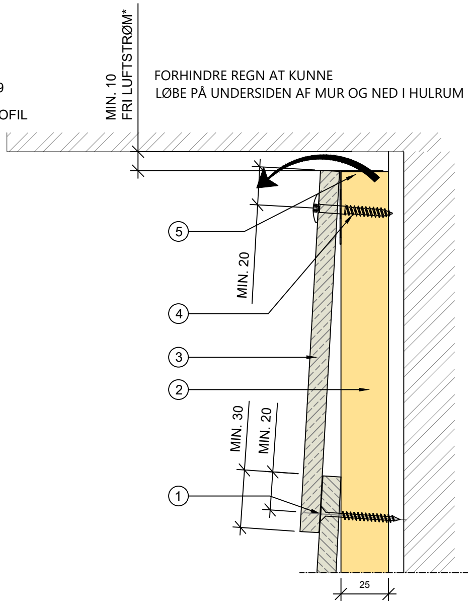
SEKTION 1:2
