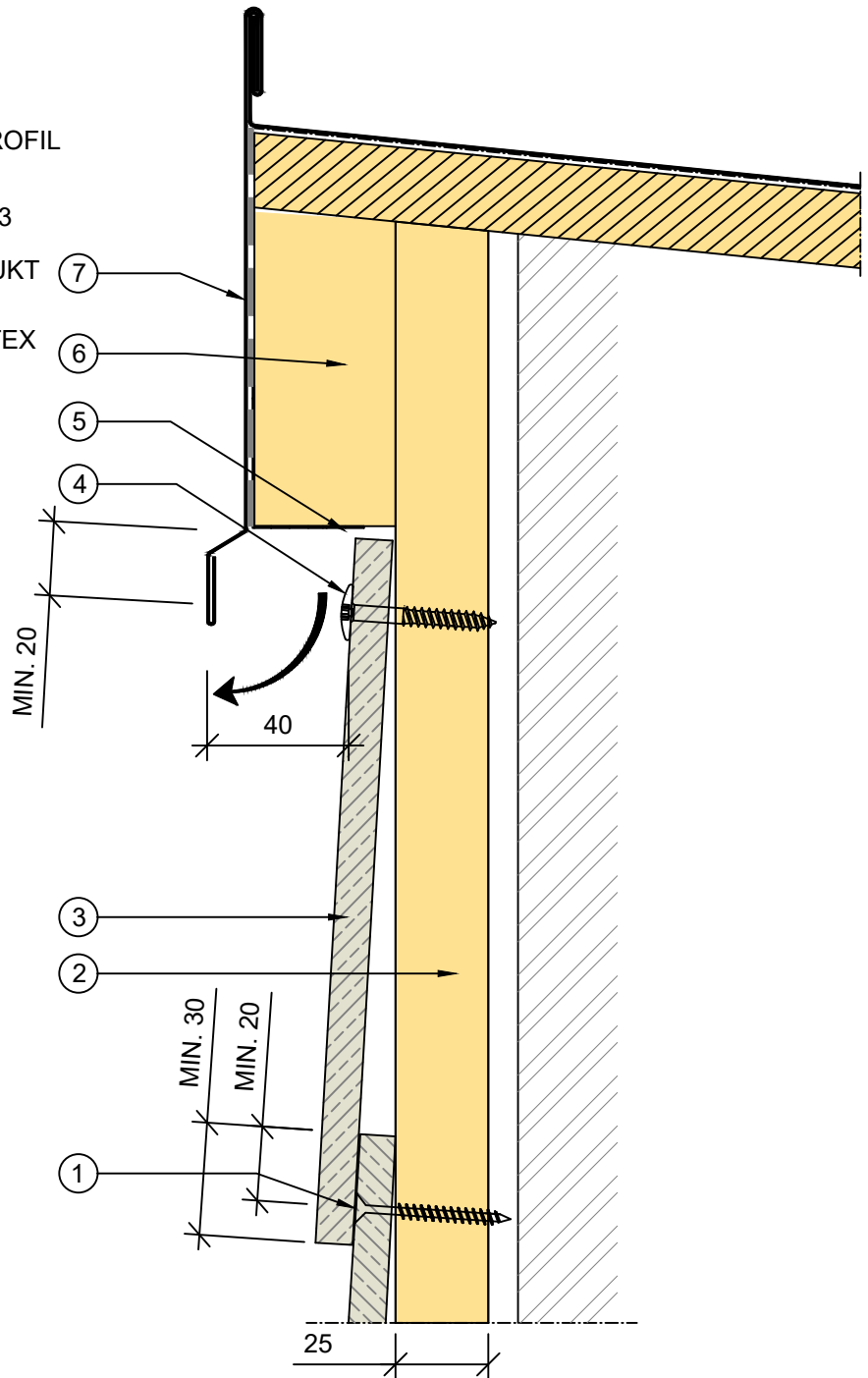
SEKTION 1:2
