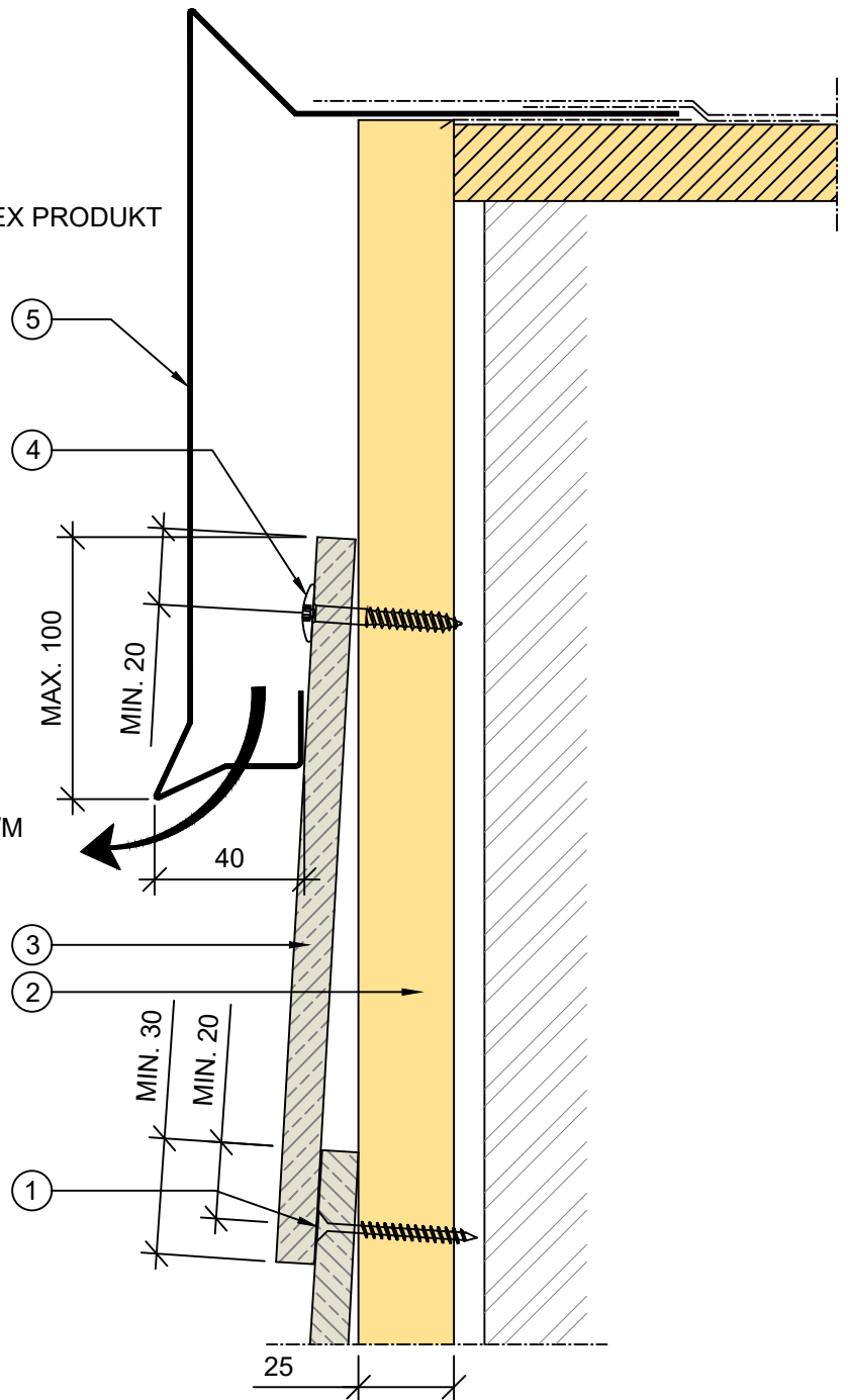
SEKTION 1:2
