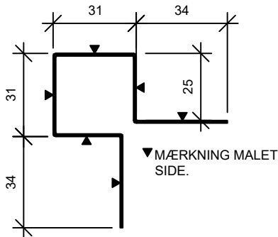
SYMMETRISK UDVENDIGT HJØRNE PROFIL
