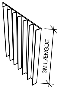
PERFORERET VENTILATIONSPROFIL [SOKKELSIKRING] ART. NR. 4017078 - UBEHANDLET ART. NR. 4017076 - SORT
