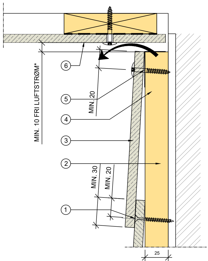
SEKTION 1:2
