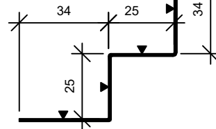
INDVENDIGT HJØRNE PROFIL
