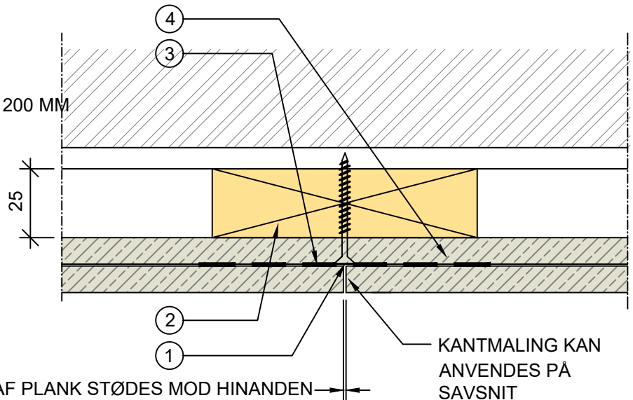
SAMMENFALDENE FUGER PLAN 1:2
