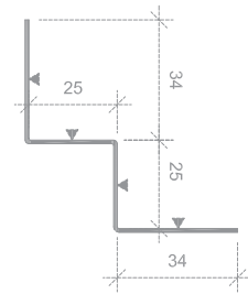
Kantprofil dubbel
