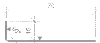
Vinkelprofil 15 mm
