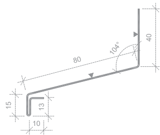
Fönsterbleck 140 mm
