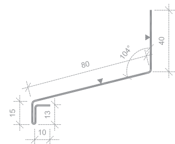
Fönsterbleck 140 mm
