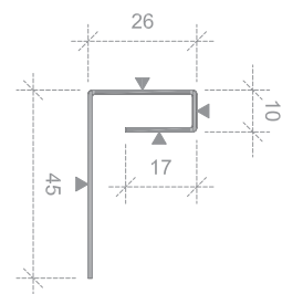
Kantprofil dubbel
