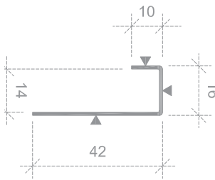
Falsbleck
