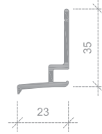
Bärprofil/dropplåt
