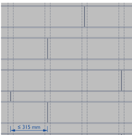
Breite und schmale Dielen, mit ungleichmäßigem Fugenversatz
