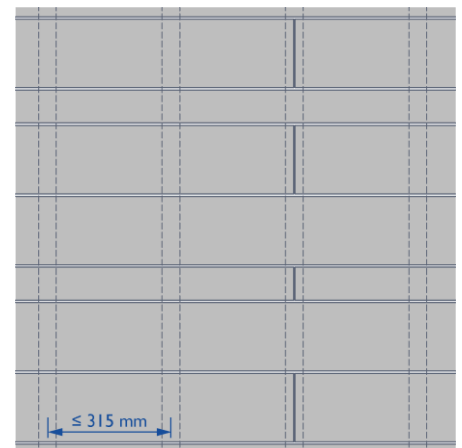
Breite und schmale Dielen, mit gleichmäßigem Fugenversatz
