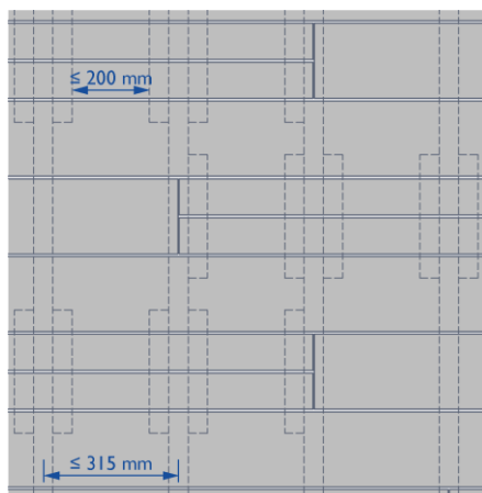
Werden 2 schmale Dielen nebeneinander verlegt, ist der lichte Abstand der Unterkonstruktion in diesem Bereich auf \leq 200 mm zu verringern
