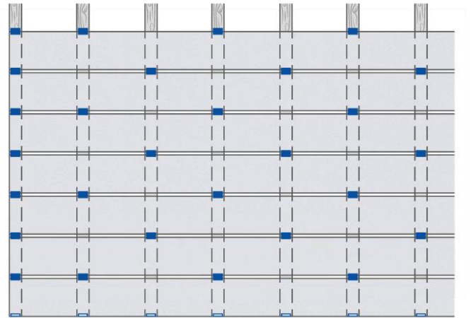
Diagonale Anordnung der Cedral Montageklammern (■) und der Cedral Start-/Endklammern (□)
