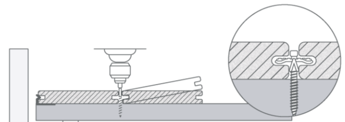
Montage der Terrassendielen mit der Cedral Montageklammer
