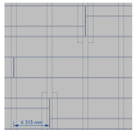
Werden breite und schmale Dielen im Stoßbereich im Wechsel verlegt, ist die Unterkonstruktion in diesem Bereich aufzudoppeln, um ausreichend Platz für die Montageklammer zu schaffen
