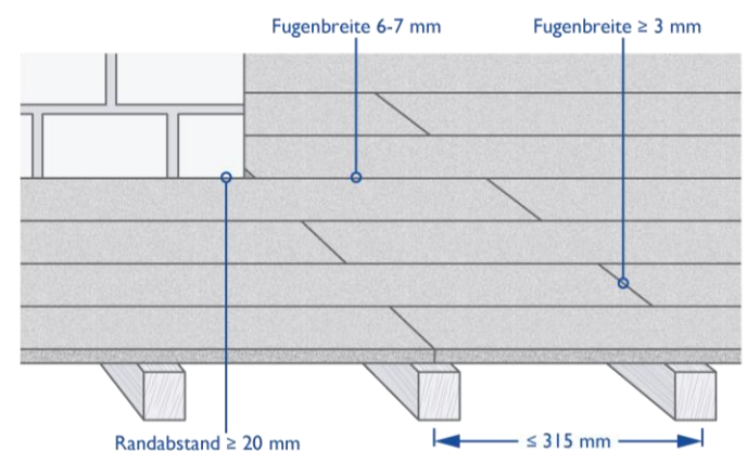
Abstände der Cedral Terrassendielen
