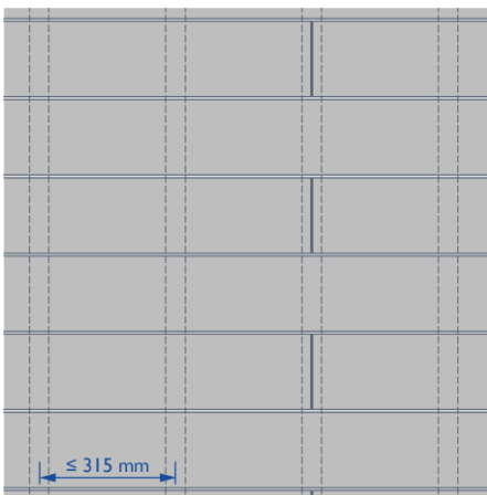
Nur breite Dielen, mit gleichmäßigem Fugenversatz
