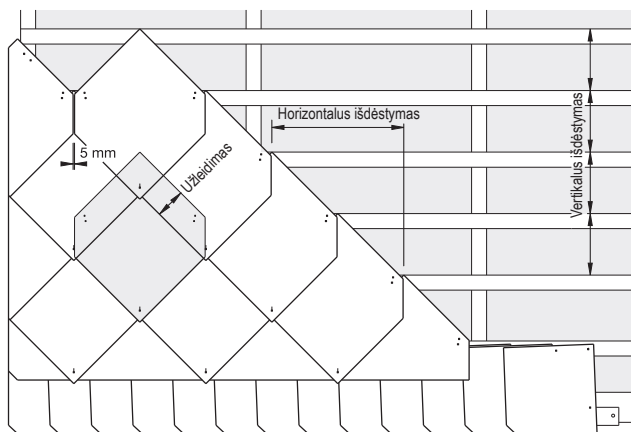
40 x 40 cm plokštelių smailiabriaunio rombo dengimas
