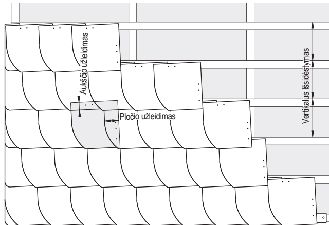
30 x 30 vokiškas fasadų dengimas su išgaubta kraštine
