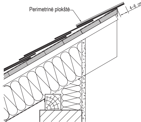
Vienšlaičio stogo kraigas dengiant ant lentų pakloto
