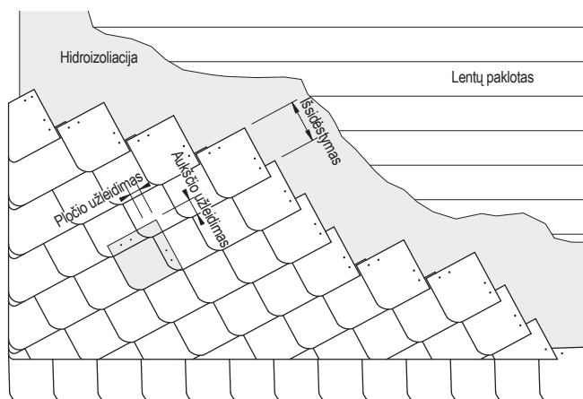
Užapvalintas dengimas naudojant 30 x 30 cm plokšteles
