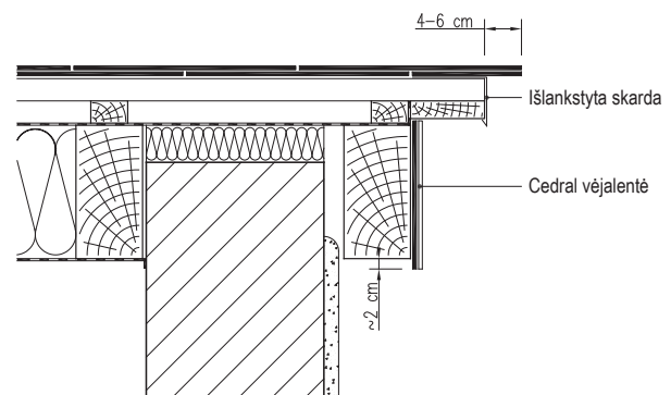
Vėjalentės įrengimas naudojant Cedral stogo plokšteles ir išlankstyta skardą
