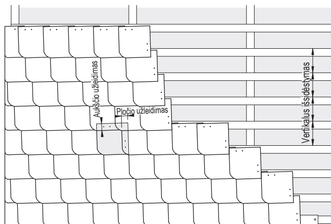
20 x 20 kilpinis dengimas užapvalintais kampais
