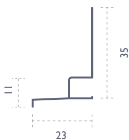
BÆREPROFIL MED VANDNÆSE
