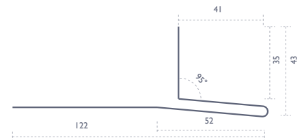
VANDNÆSE
