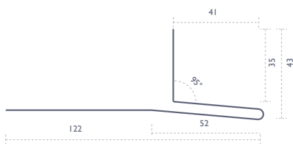
VANDNÆSE
