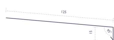
SÅLBÆNK
