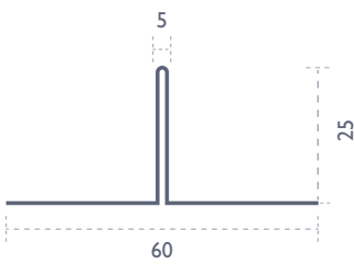
SAMLEPROFIL
