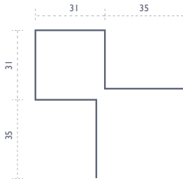
UDVENDIGT HJØRNE SYMMETRISK
