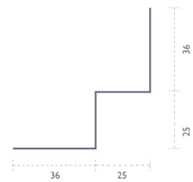
INDVENDIGT HJØRNE
