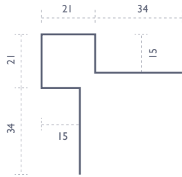
UDVENDIGT HJØRNE SYMMETRISK FACADE
