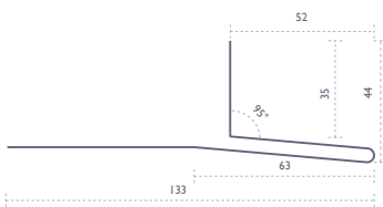
VANDNÆSE
