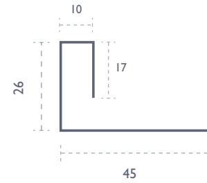
DOBBELT ENDEKANT
