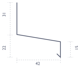
VANDNÆSE (TIL MONTAGE PÅ VÆG)
