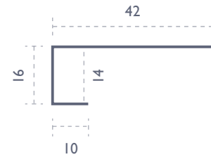
ENKEL ENDEKANT
