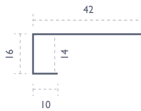
ENKEL ENDEKANT
