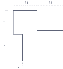
UDVENDIGT HJØRNE ASYMMETRISK
