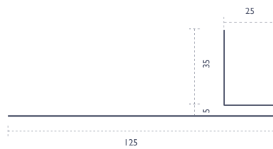
SIDEINDDÆKNING
